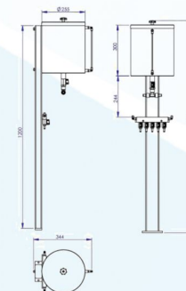
ALÜMİNYUM VE KOMPOZİT PROFİLLER İÇİN PRİMER ÜNİTESİ PRİMER UNIT FOR ALUMINIUM AND COMPOSITE PROFILES
